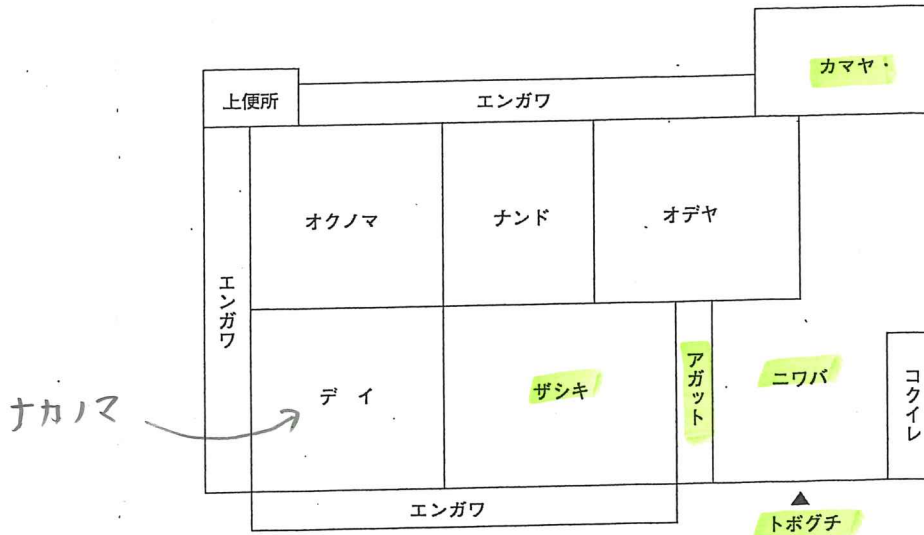
図2-28 右勝手の間取り
