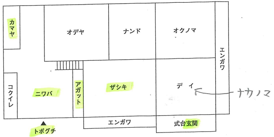
図2-29 左勝手の間取り
